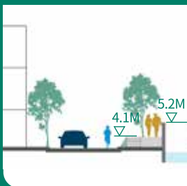
局部抬高人行道岸线剖面图
