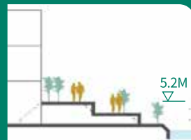
设置两级防汛墙岸线剖面图
